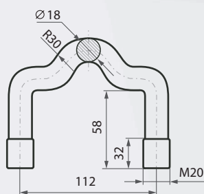
Обойма гнутая
